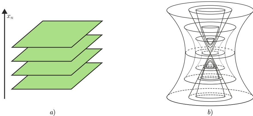
Рис. 1.1. Пример множеств уровня в окрестности регулярной и критической точки
